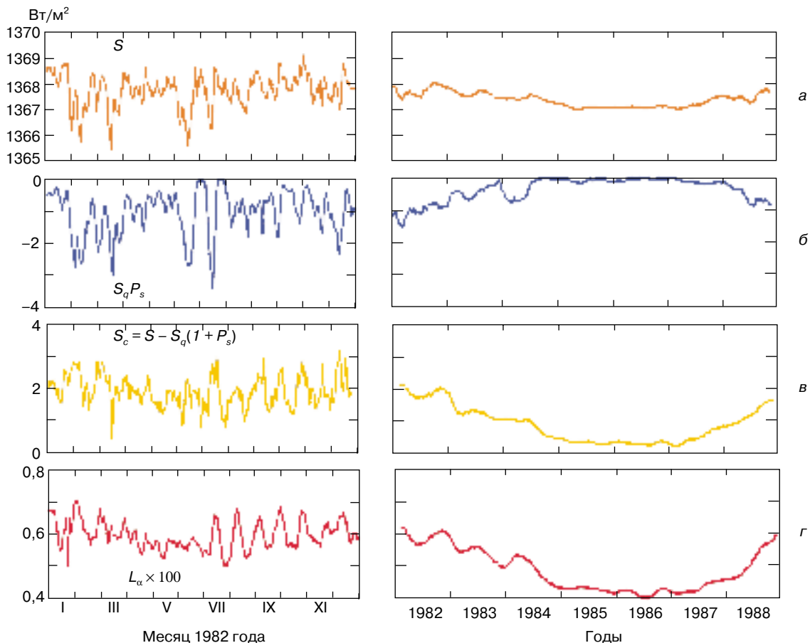
Рис. 3. Вариации среднесуточных (слева) и осредненных по 81-дневным интервалам (справа) величин: a – полная солнечная радиация S ; b – блокировка солнечной радиации пятнами S_q P_s ; c – остаточная солнечная радиация S_c = S - S_q(1 + P_s) ; d – интенсивность солнечной радиации в L_\alpha -свете.
