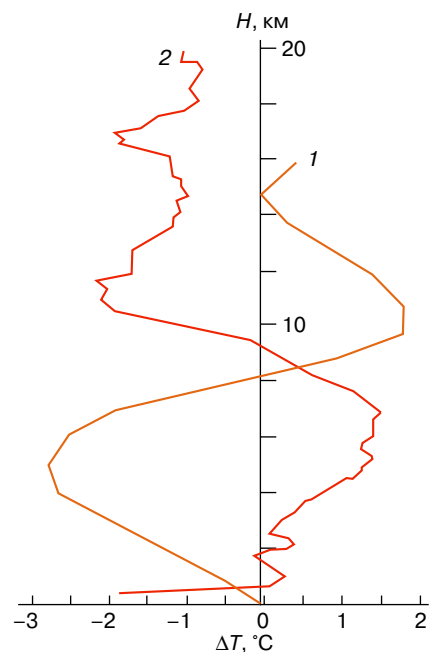
Рис. 5. Высотный профиль отклонений температуры воздуха \Delta T от “спокойного” уровня во время всплесков СКЛ (кривая 1) и форбуш-понижений (кривая 2).
